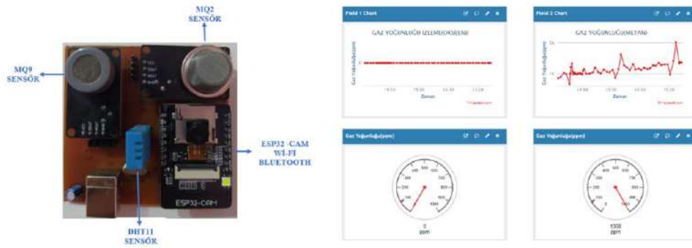
Şekil 2. a) Ölçüm Düğümü Prototipi b) Nesnelerin İnterneti Sunucusu Örnek
